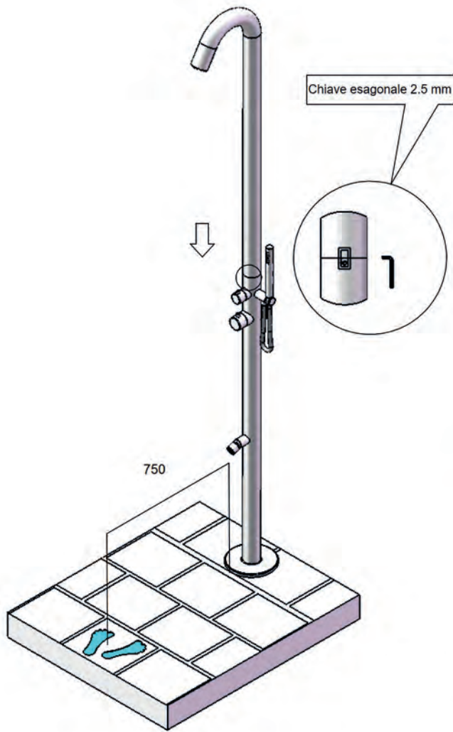
La C-BOX con i tubi dell'acqua calda e fredda è nascosta sotto il pavimento.
